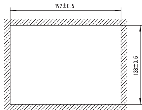
开孔尺寸
