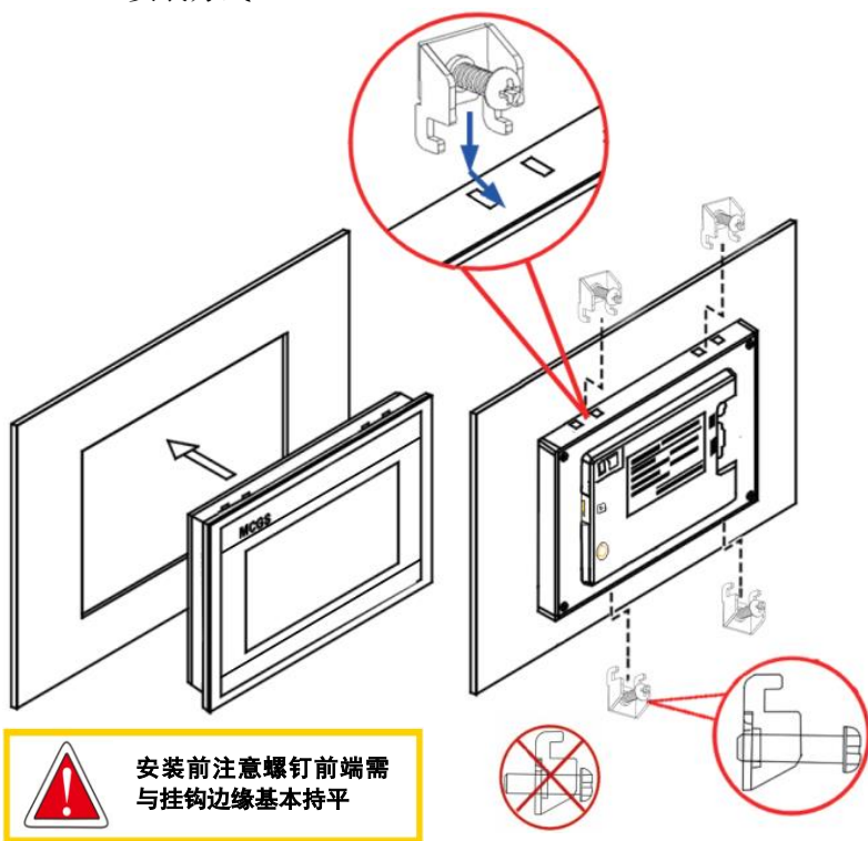
挂钩安装
