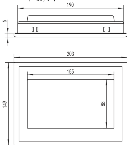
外形尺寸
