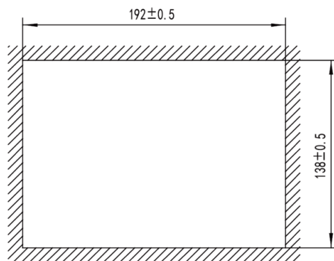
开孔尺寸
