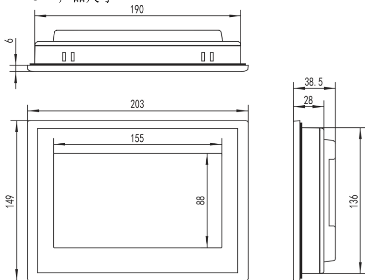
外形尺寸
