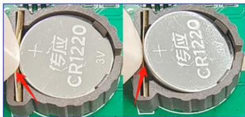
拆卸电池
