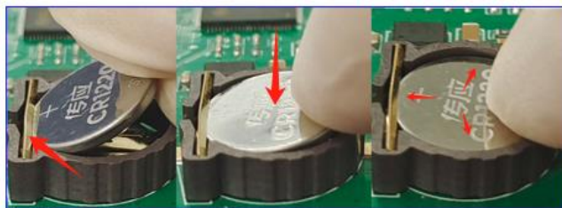
安装电池
