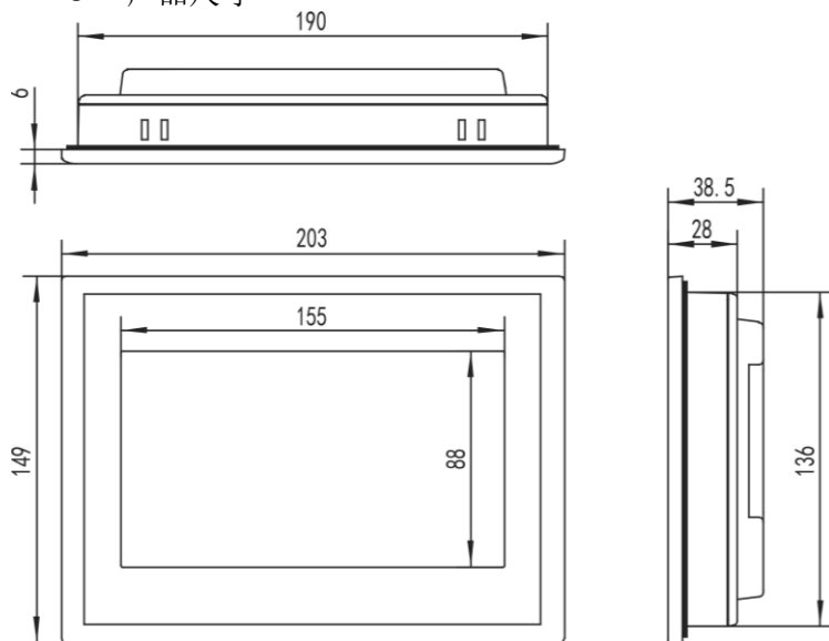
外形尺寸
