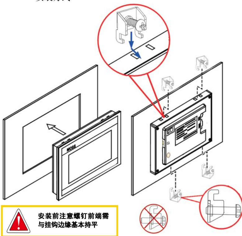
挂钩安装
