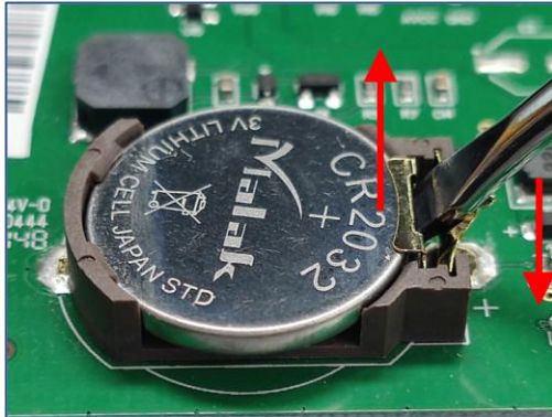
拆卸电池
