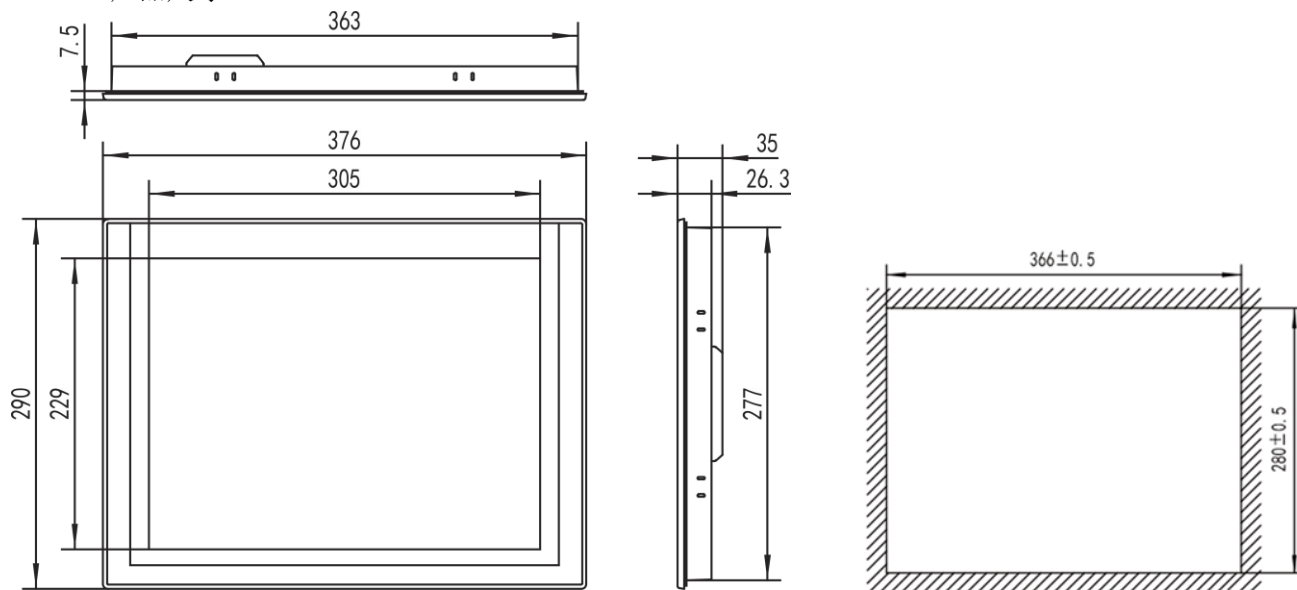
外形尺寸
