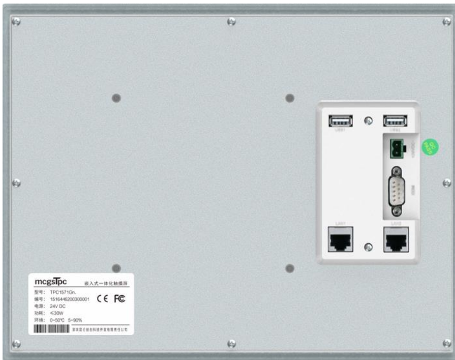
底视图
