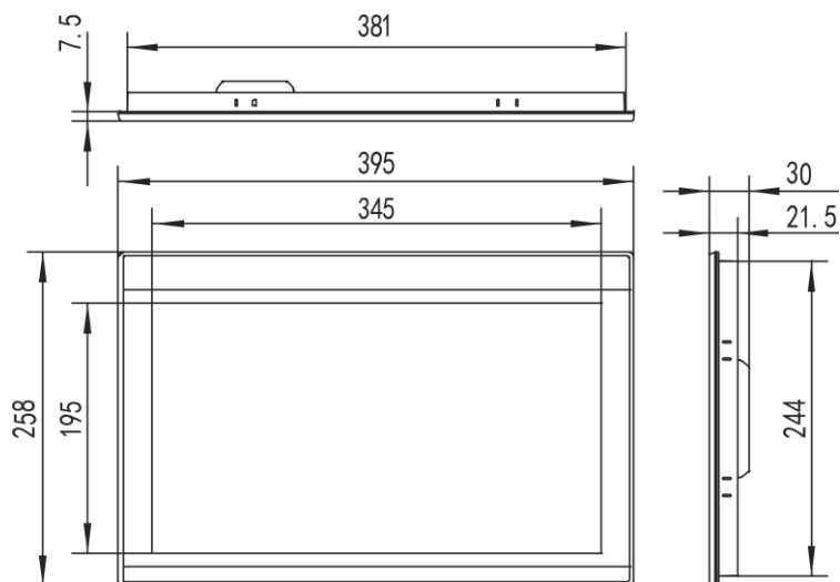
外形尺寸
