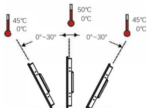
安装角度
