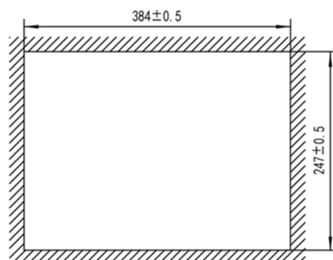
开孔尺寸
