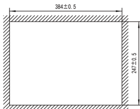
开孔尺寸
