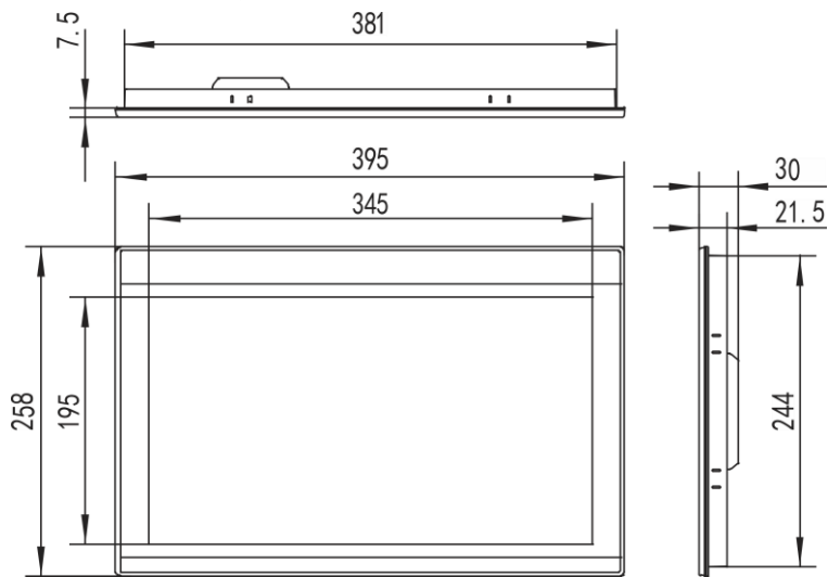
外形尺寸
