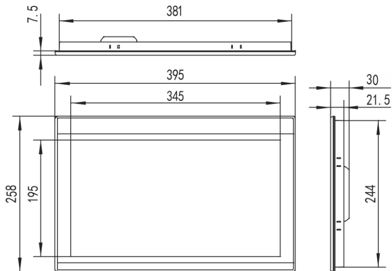
外形尺寸
