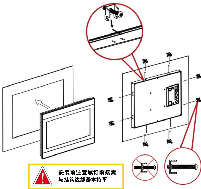
挂钩安装
