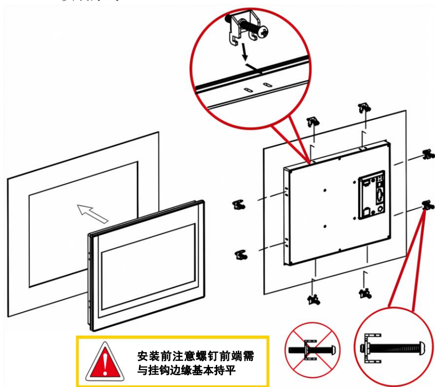
挂钩安装
