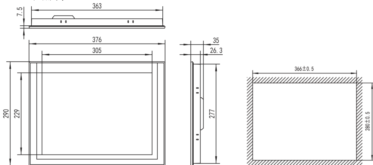
外形尺寸
