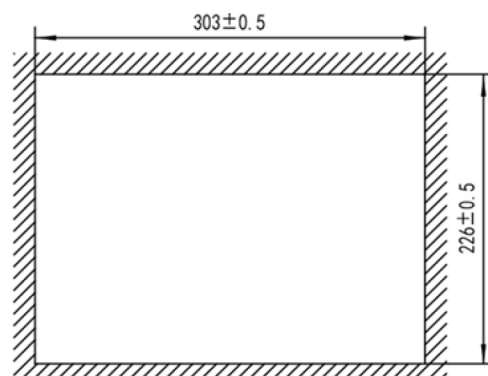
开孔尺寸
