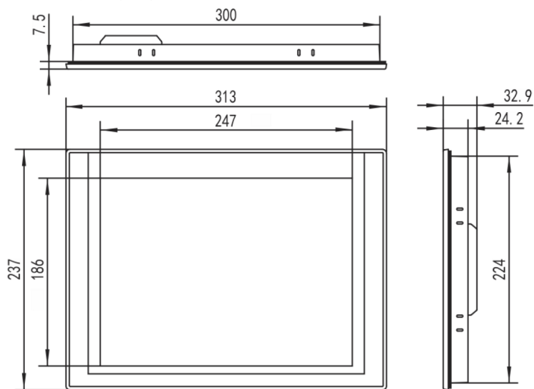
外形尺寸
