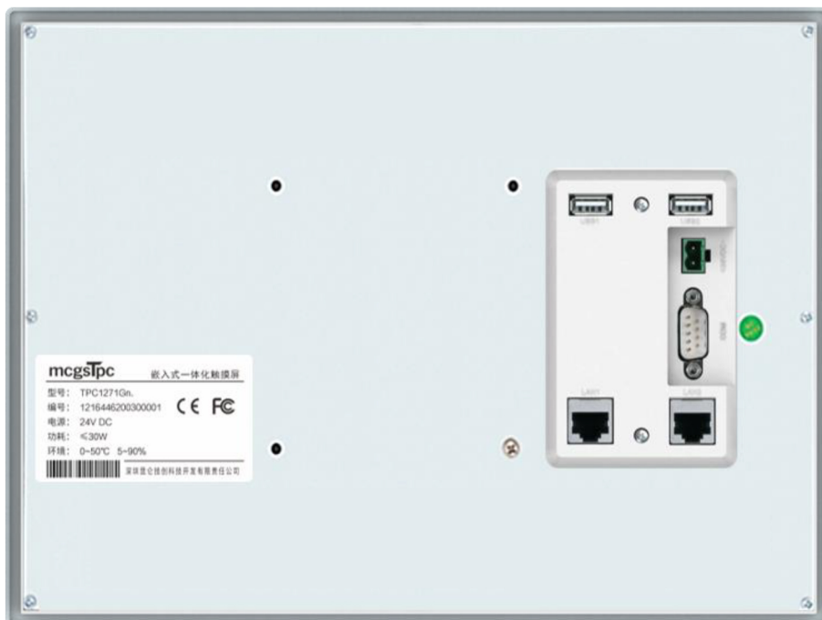
底视图
