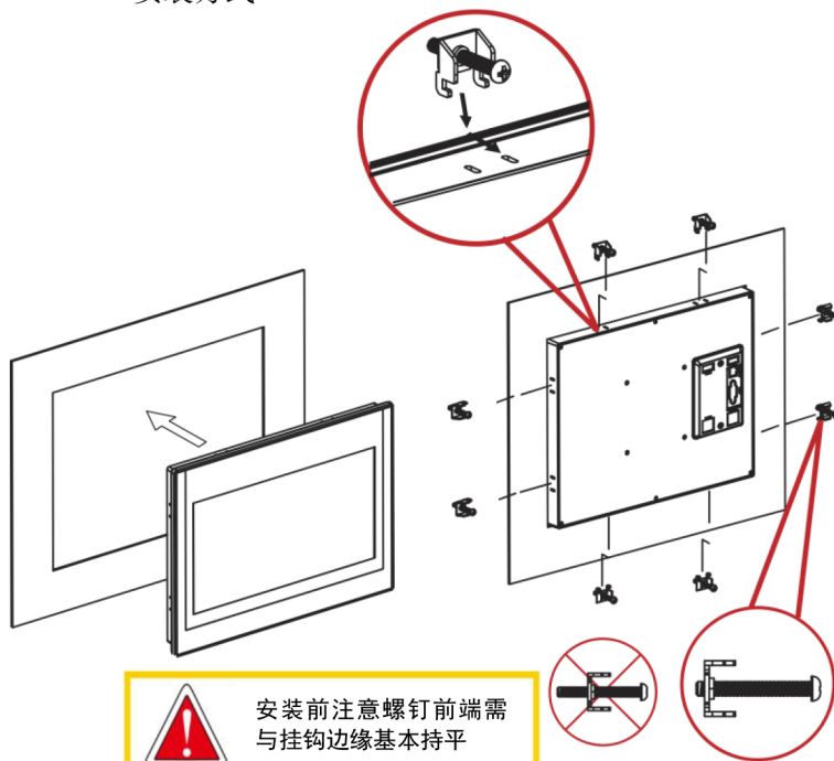
挂钩安装
