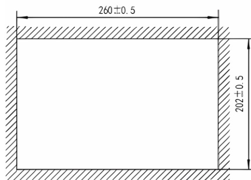
开孔尺寸
