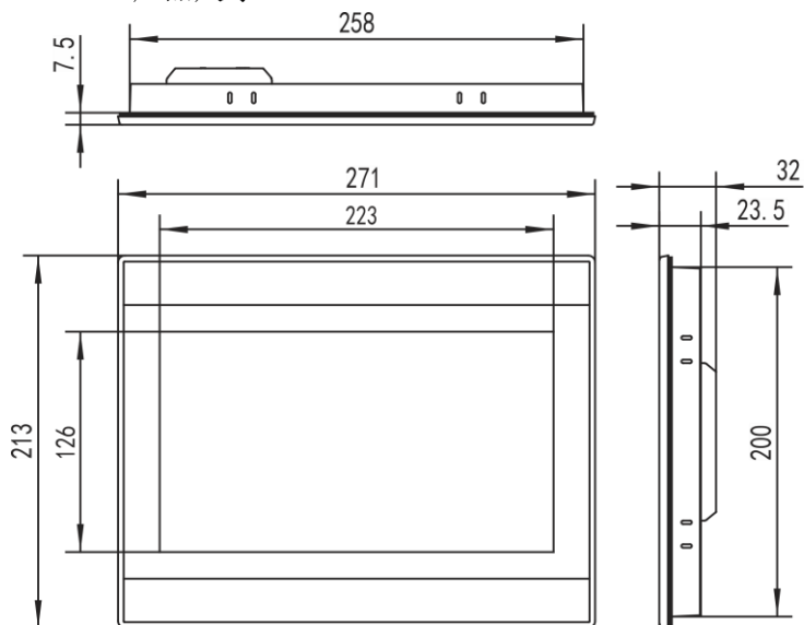
外形尺寸
