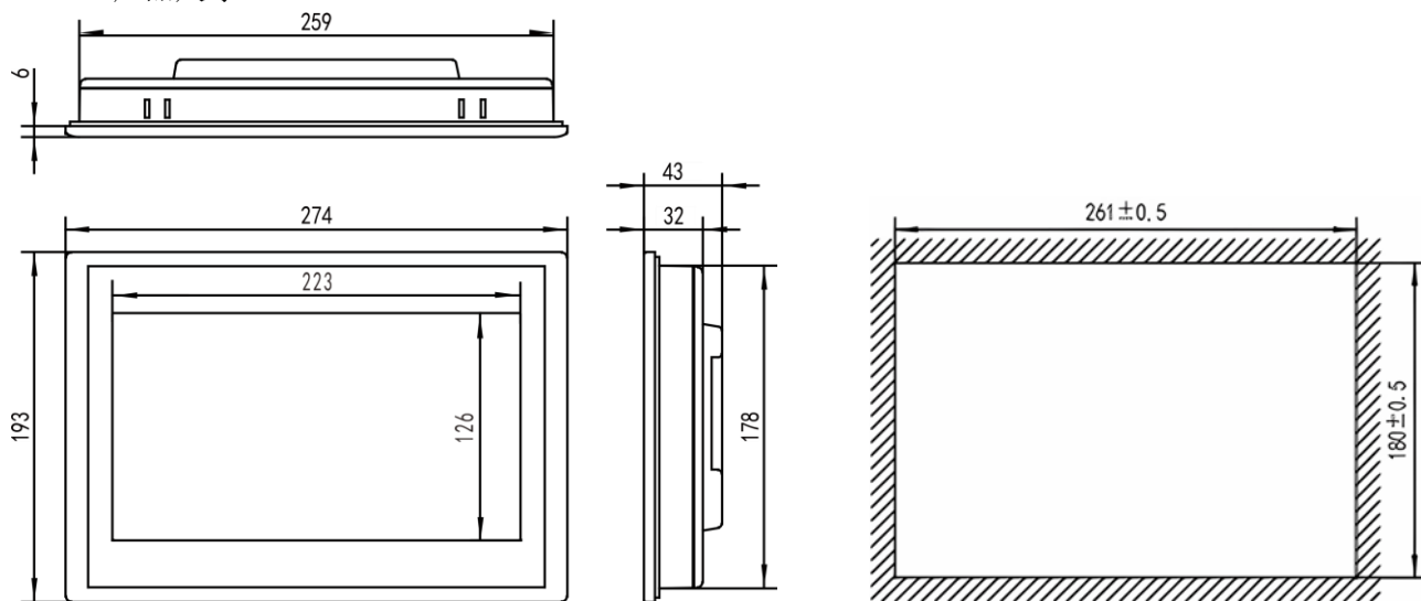
外形尺寸
