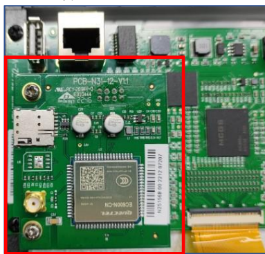
取下扩展版
