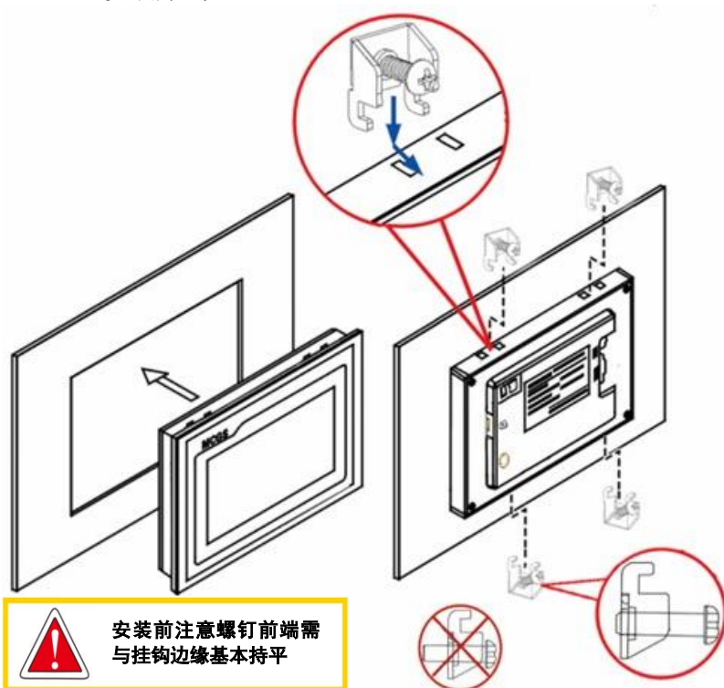
挂钩安装
