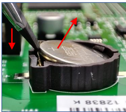
拆卸电池
