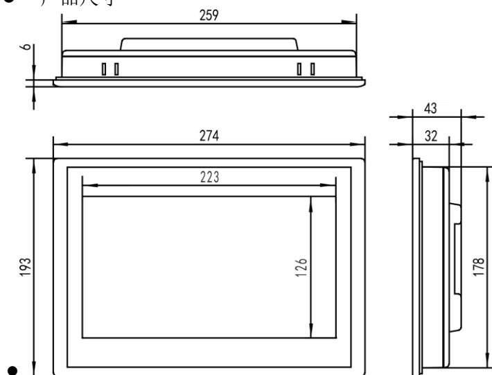
外形尺寸
