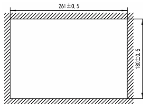
开孔尺寸
